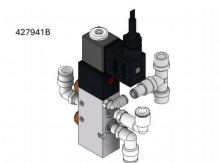
427941B SET PULLER OPEN/CLOSE SET ABZUG AUF/ZU 4V210ex-06-DC24V
