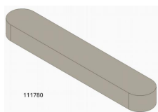
111780 feather key DIN 6885 A18x11x110 Passfeder 18h9x 11h11x110 DIN6885A C45K
