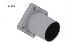
114803 linear ball bearing w. square flange Ø16 Linearkugellager mit Vierkantflansch Ø16
