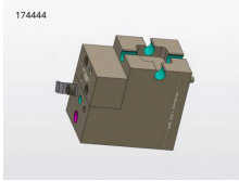
174444 RED.PCE heater block unit M12x1 Ø14 RED.PCE Heizblockeinheit M12x1 Ø14
