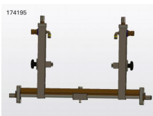
174195 RED.PCE stand for 2 bars width=415 RED.PCE-Verstell-EH Leiste 2 Turm B=415
